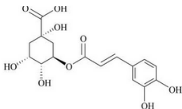
Figure 20 Acide chlorogénique
